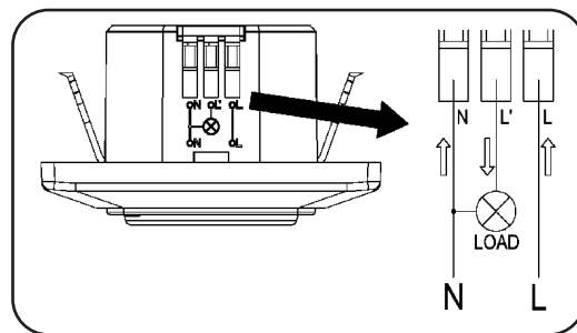
Fig.3: Conexión del sensor.
