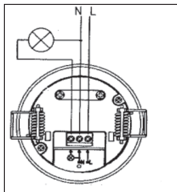
Fig. 3 Conexión
