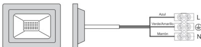
Diagrama de conexión
