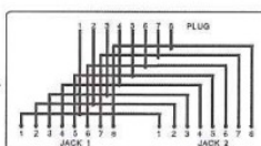
Connection diagram Diagrama de conexión
