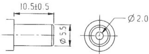
Conector macho para mod. 15.479
